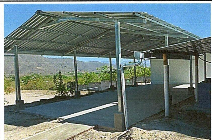
Foto 3: Finalización de la estructura tipo pórtico e instalación de lámina troquelada calibre 26 en salón de reuniones y mejoramiento de piso
