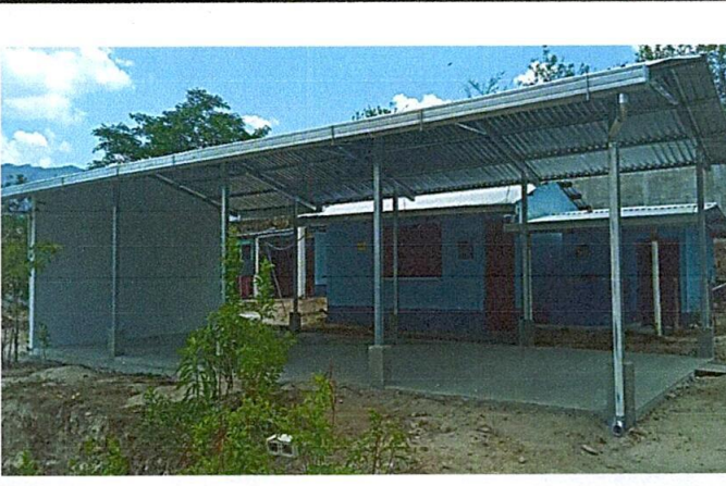
Foto 4: Finalización de la estructura tipo pórtico e instalación de lámina troquelada calibre 26 en salón de reuniones y mejoramiento de piso
