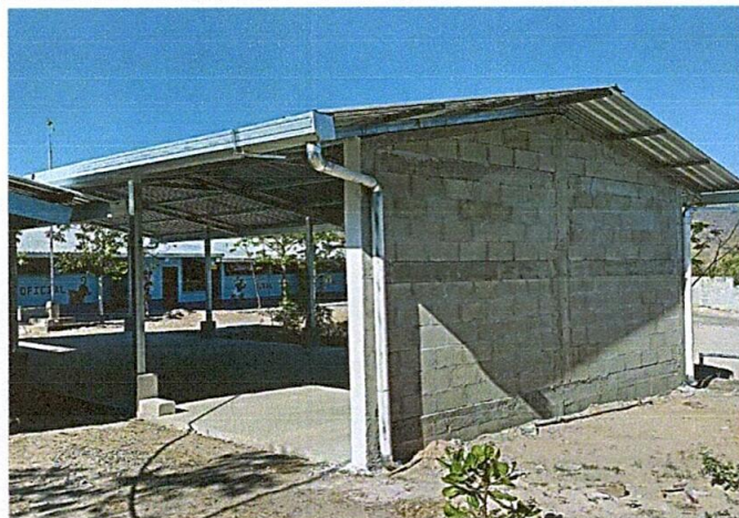
Foto 2: Finalización de la estructura tipo pórtico e instalación de lámina troquelada calibre 26 en salón de reuniones y mejoramiento de piso
